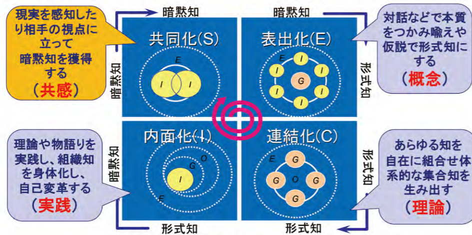
図1 SECIモデル
